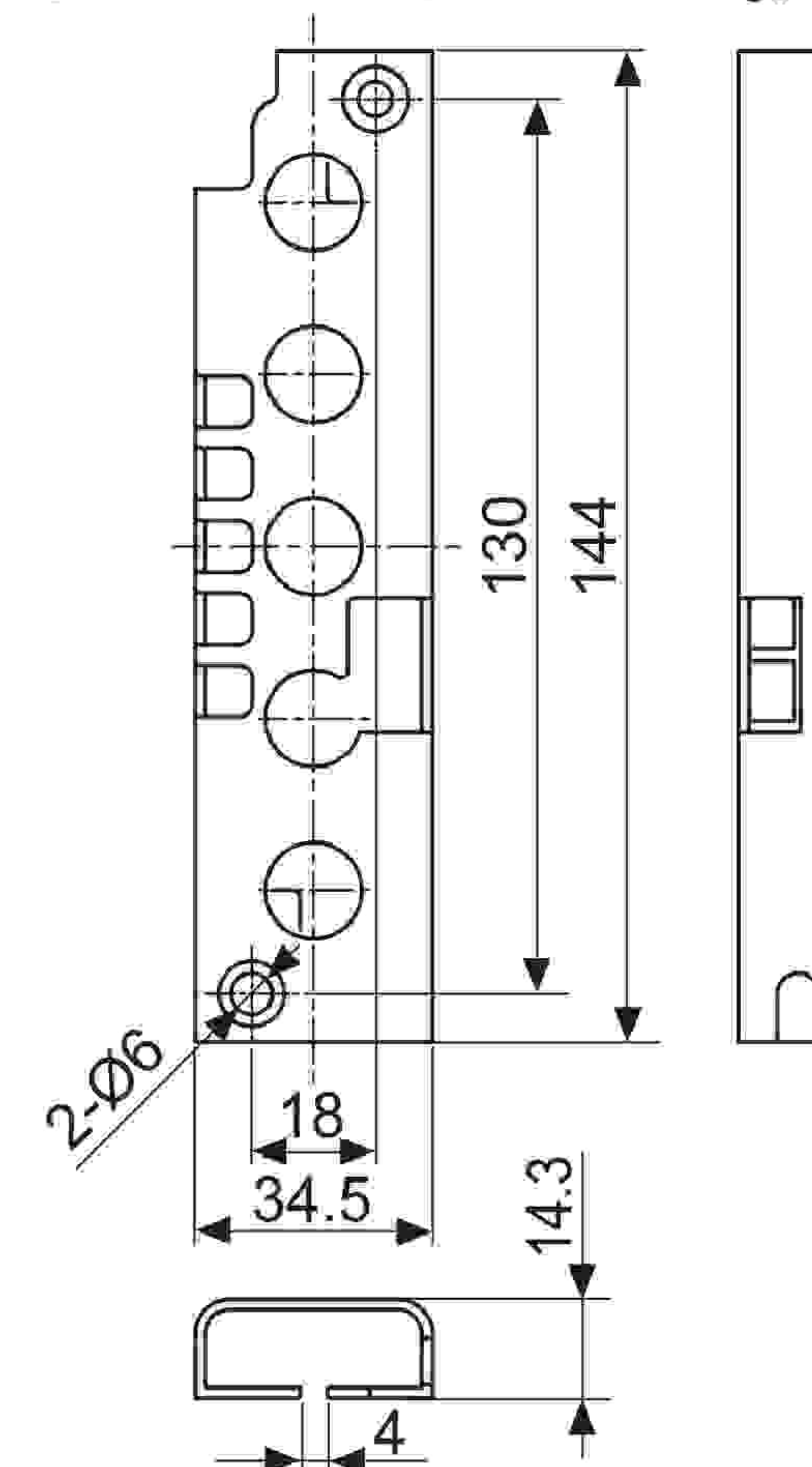
* براکت محافظ (BK-BWPK-P)
