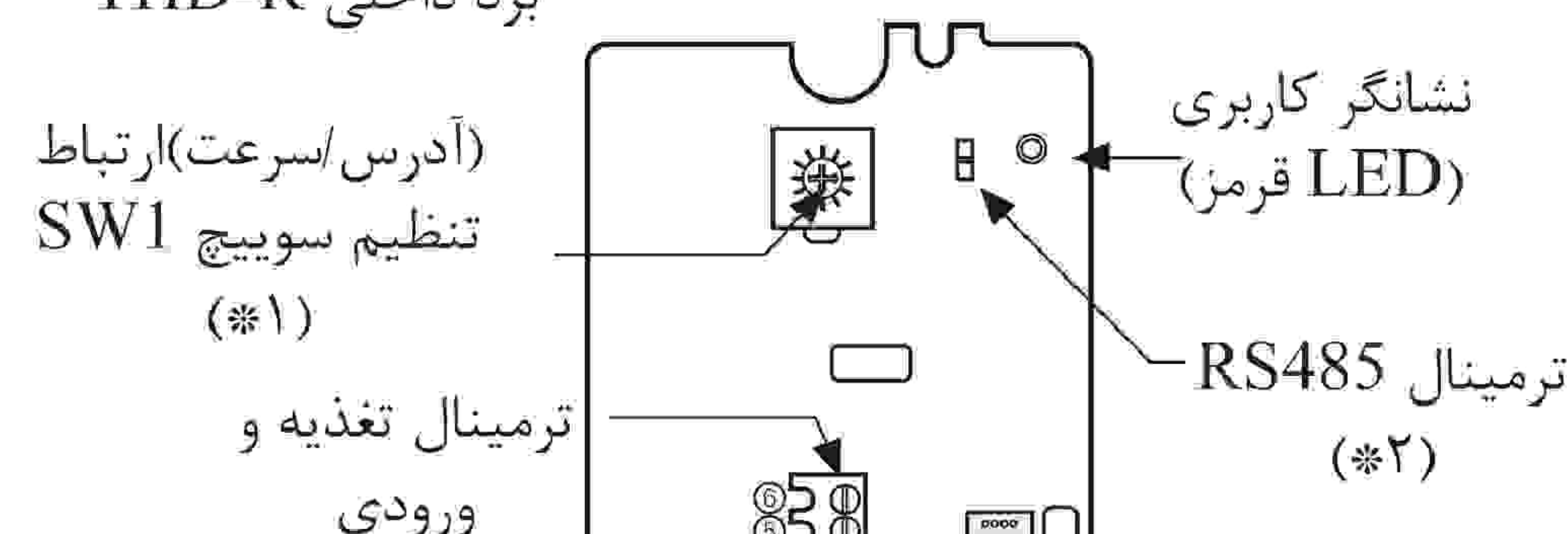
برد داخلی THD-R
